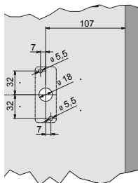
RFID-Leser L043-A02 ohne Zwischenlage
