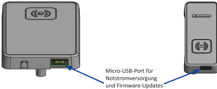
RFID-Leser L033-A01
