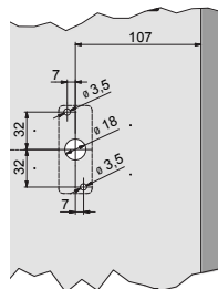
RFID-Leser L043-A02 mit Zwischenlage
