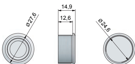
Fingerprint module / Lector de huellas
