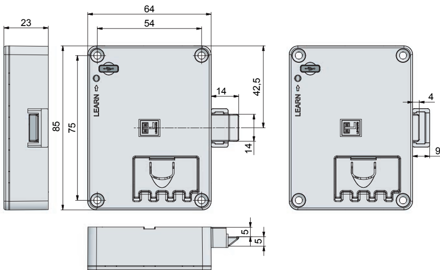
Lock M410 pro / Cerradura M410 pro
