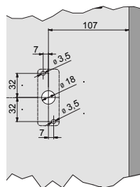
RFID-Leser L033-A02 mit Zwischenlage
