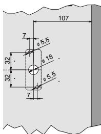
RFID-Leser L033-A02 ohne Zwischenlage
