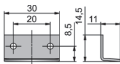
Ergot de verrouillage 3011
