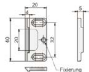
Schließwinkel
