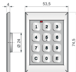
M400 Tastatur
