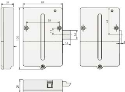
M400 Elektronik
